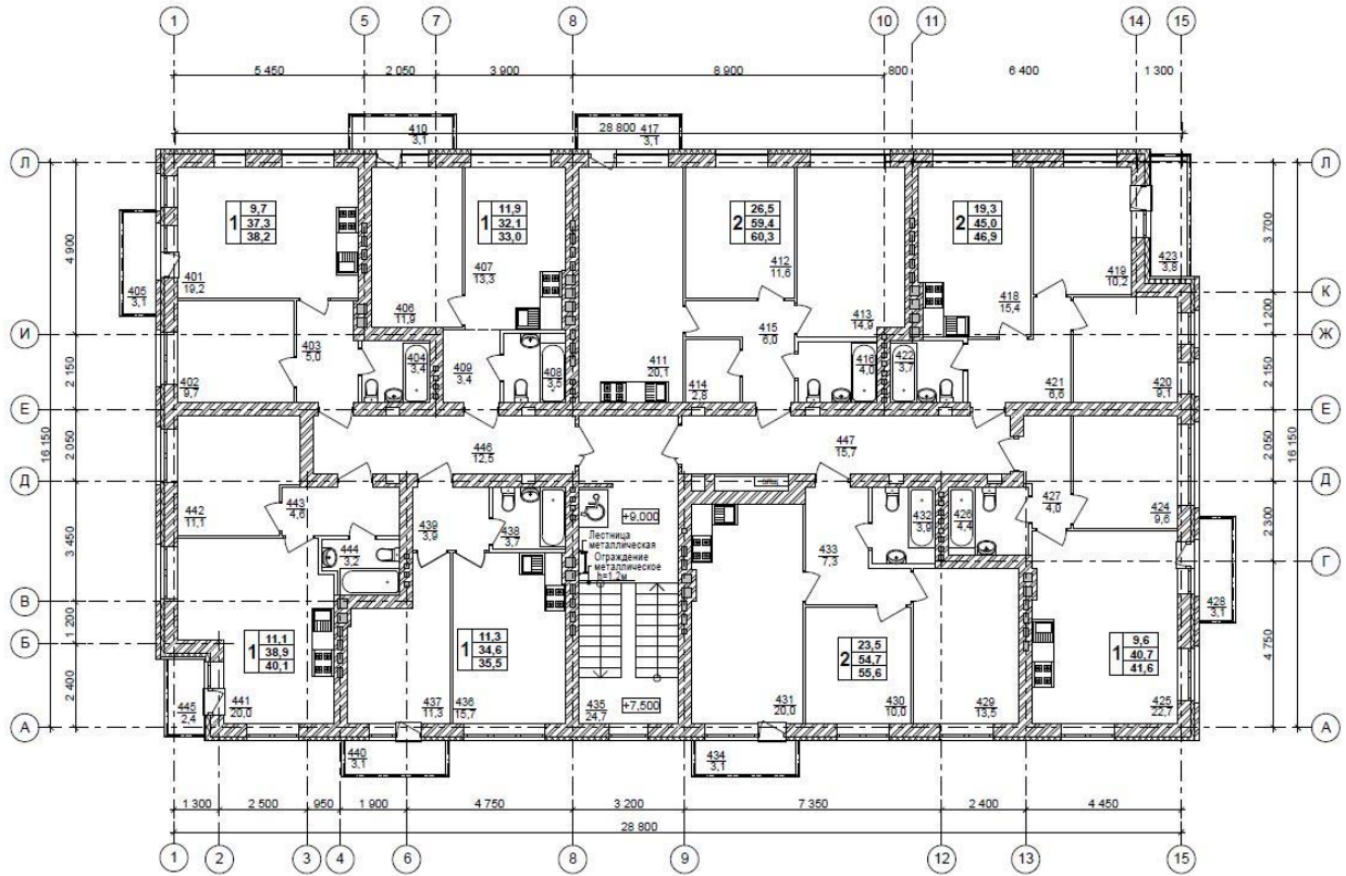
План 4 этажа
