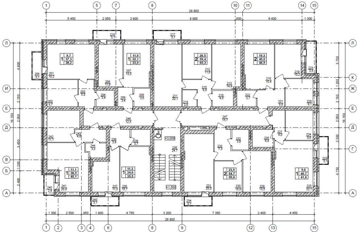
План 2 этажа
