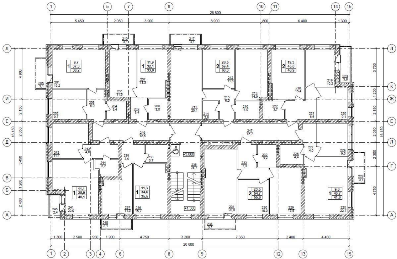
План 2 этажа
