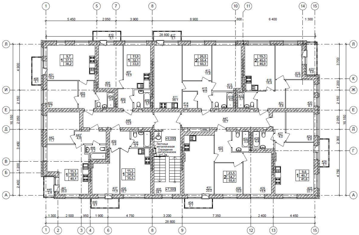
План 4 этажа
