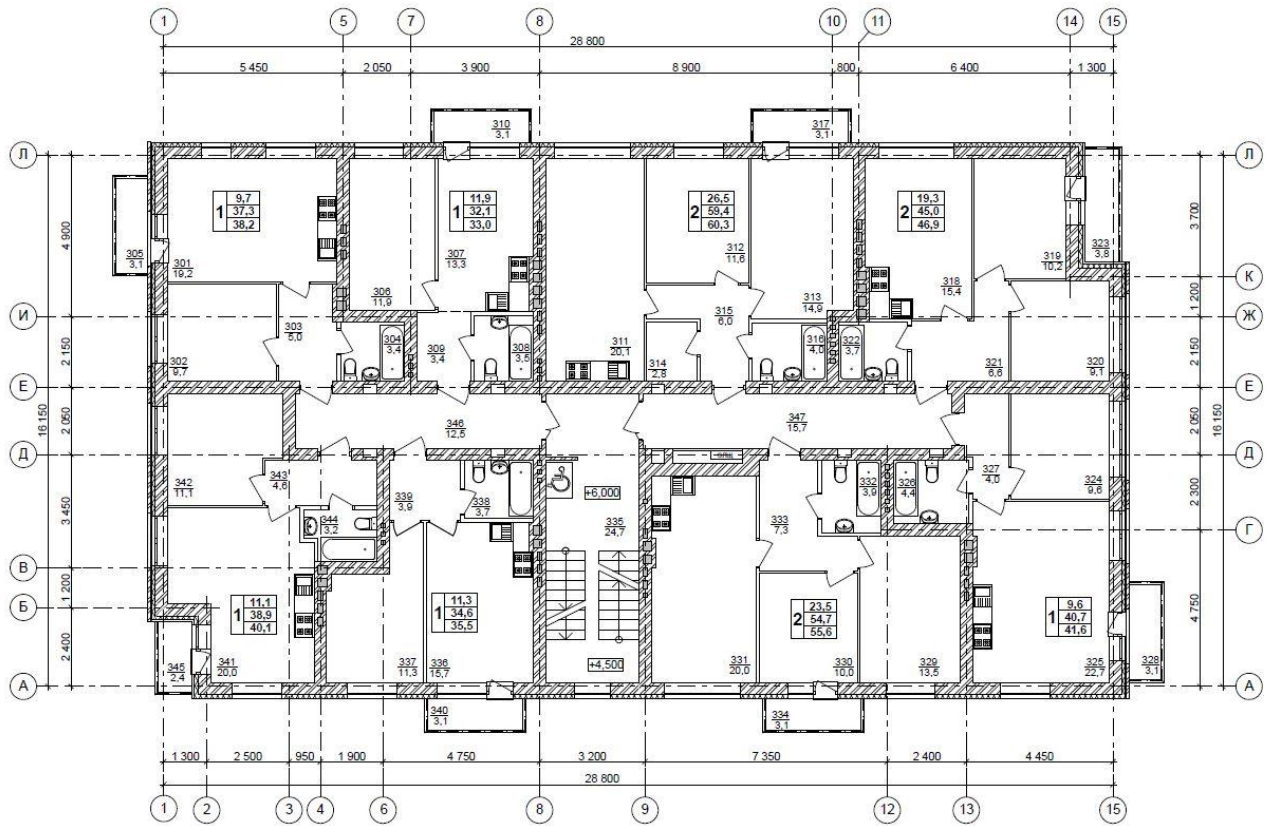
План 3 этажа
