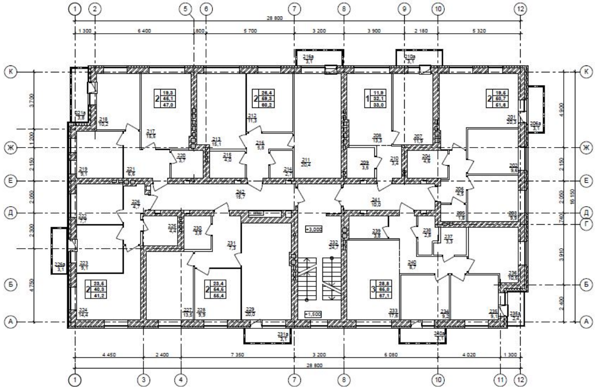
План 2 этажа
