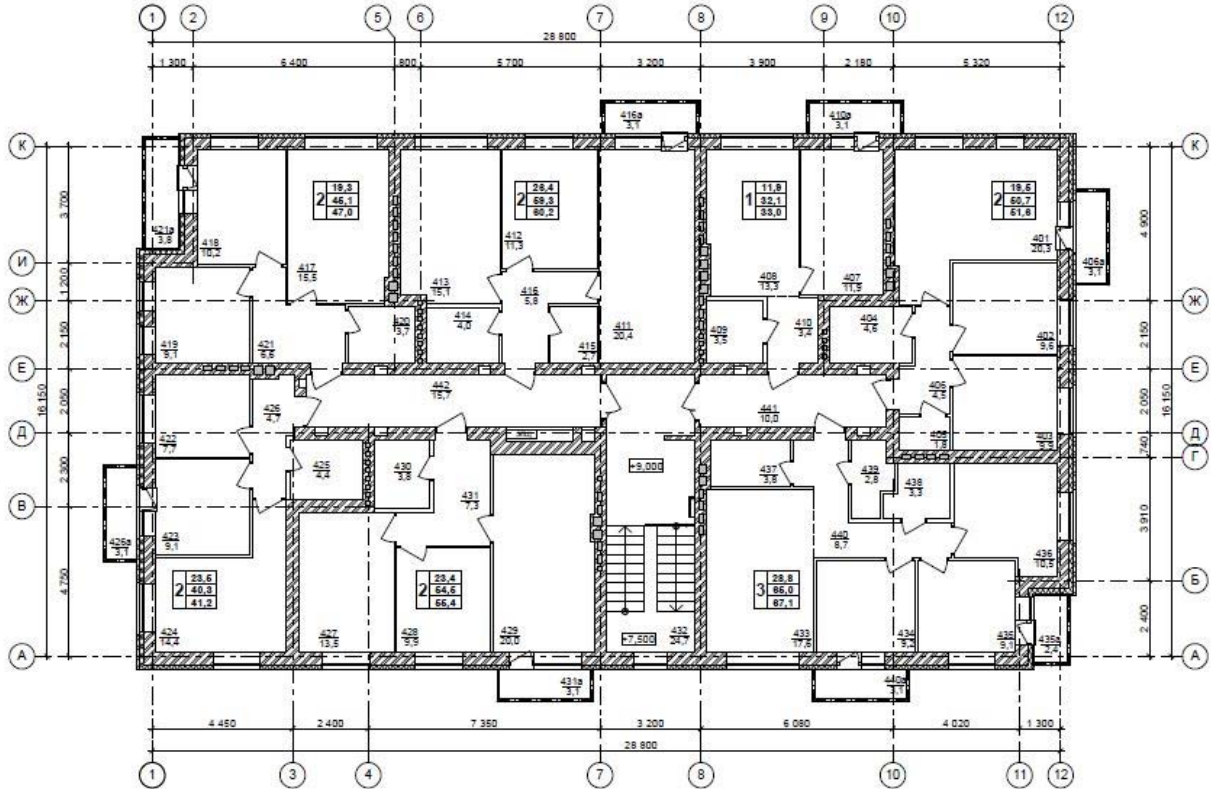
План 4 этажа
