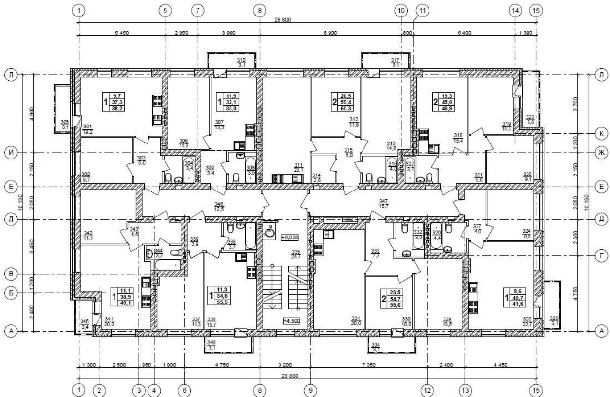
План 3 этажа
