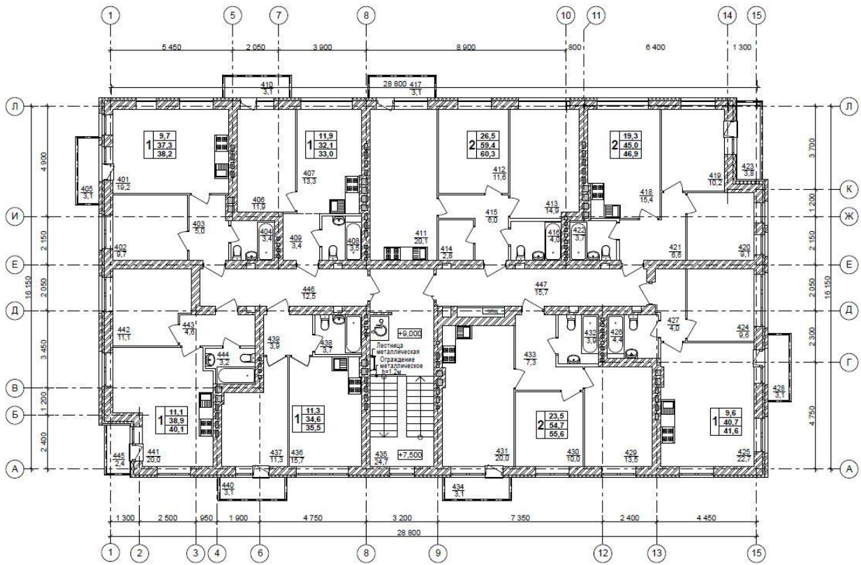
План 4 этажа
