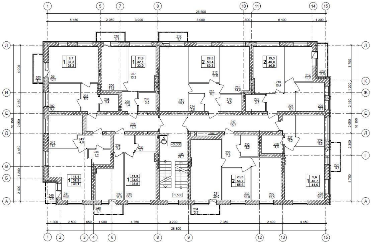
План 2 этажа
