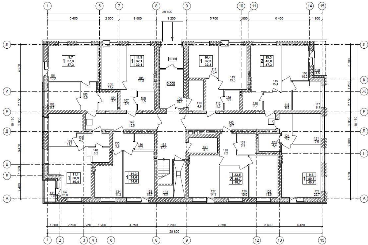
План 1 этажа
