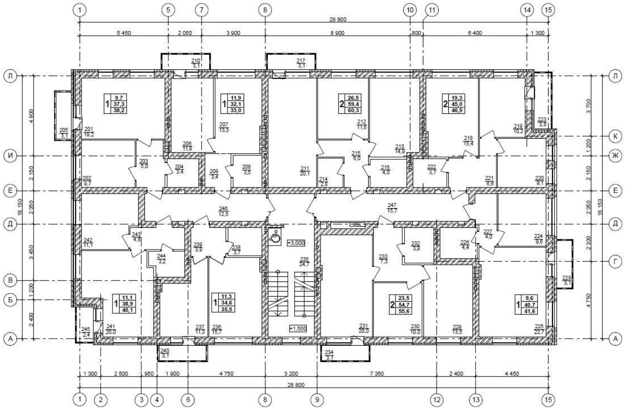
План 2 этажа
