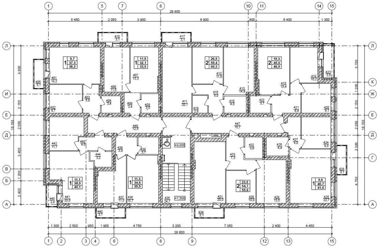
План 4 этажа
