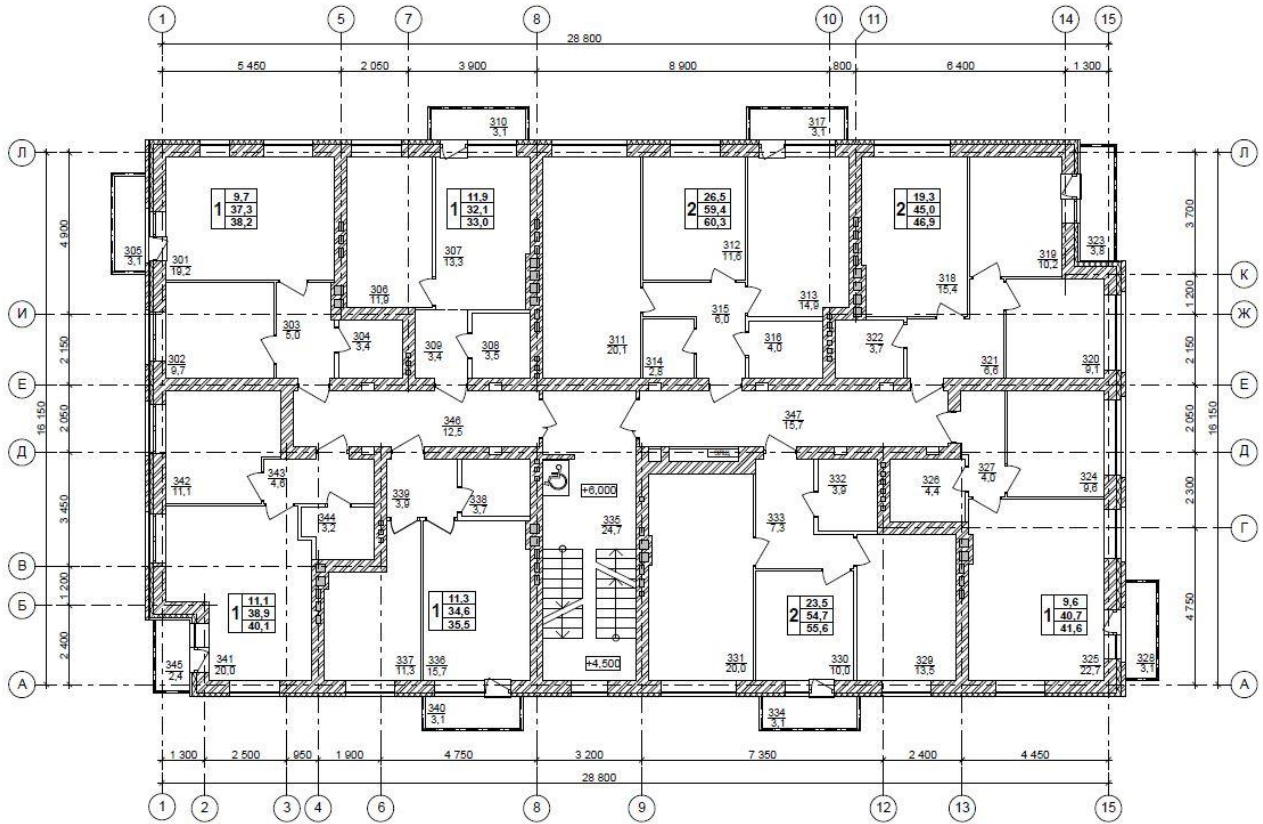
План 3 этажа
