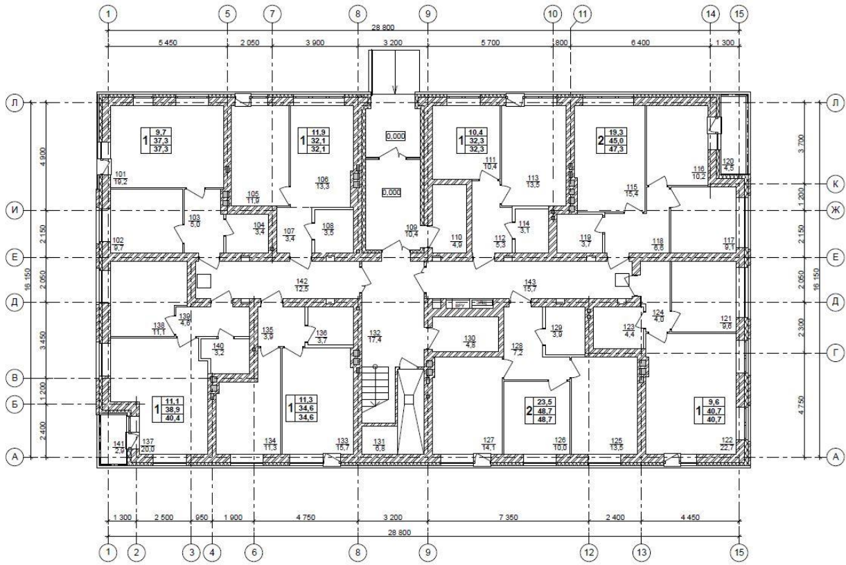
План 1 этажа
