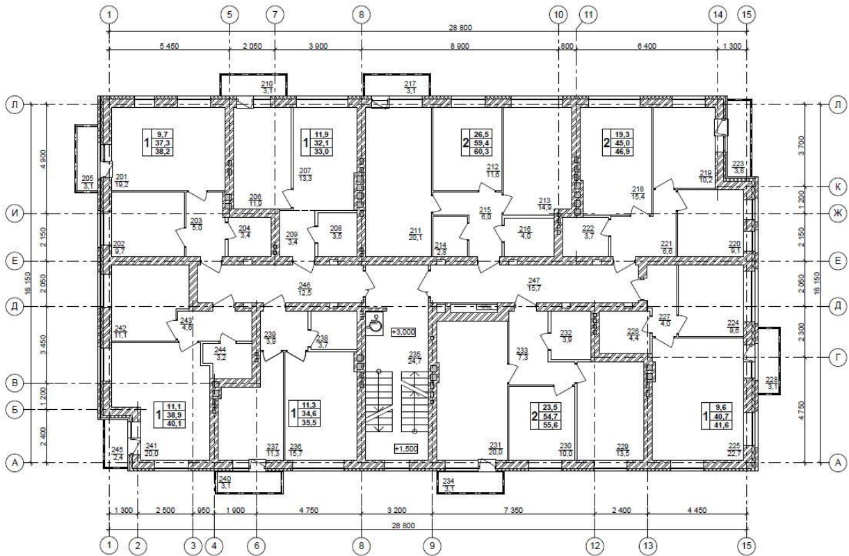
План 2 этажа
