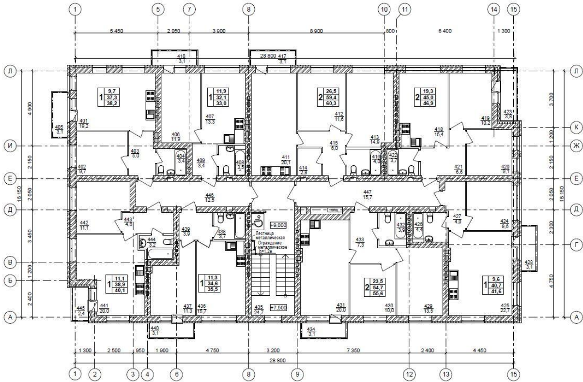
План 4 этажа
