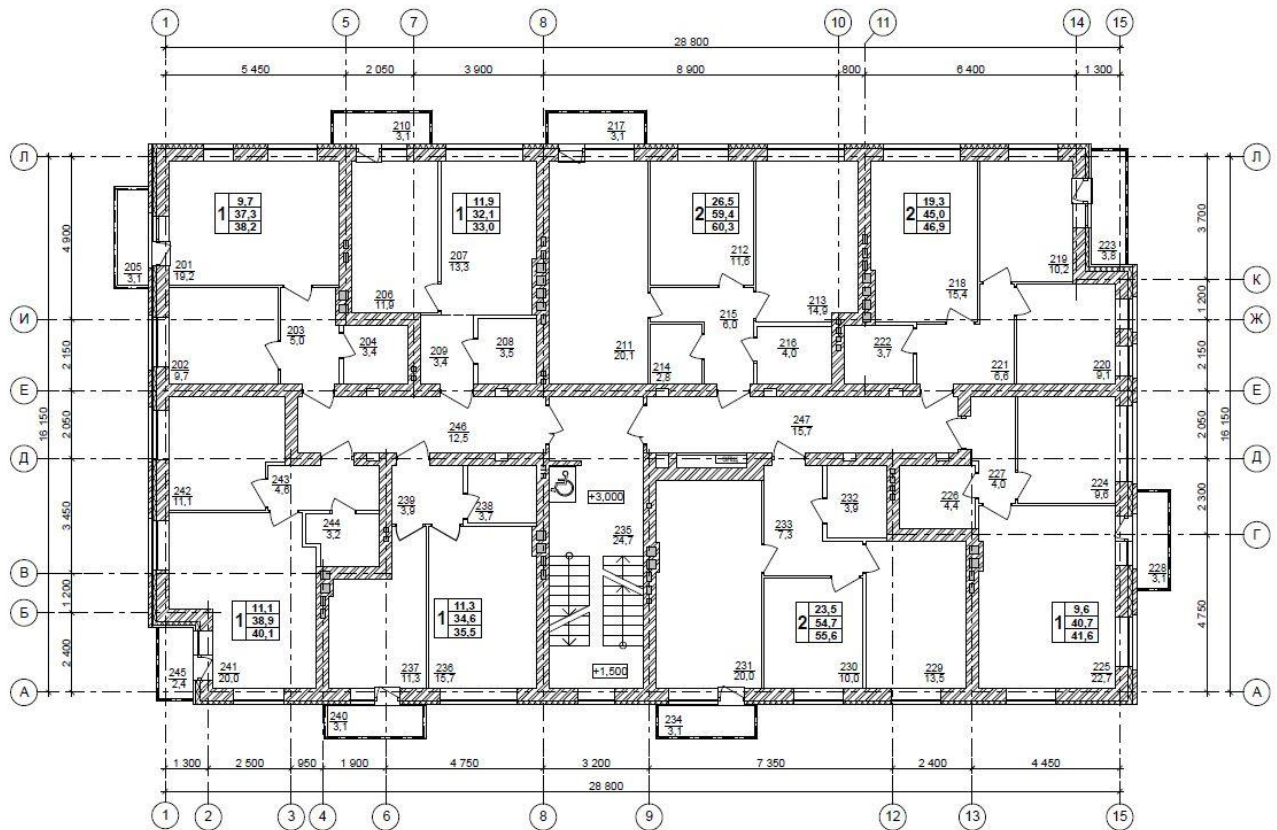
План 2 этажа
