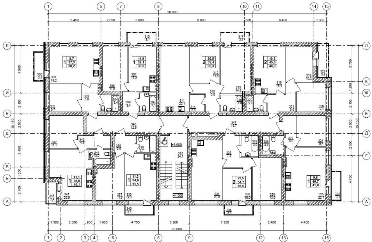
План 3 этажа
