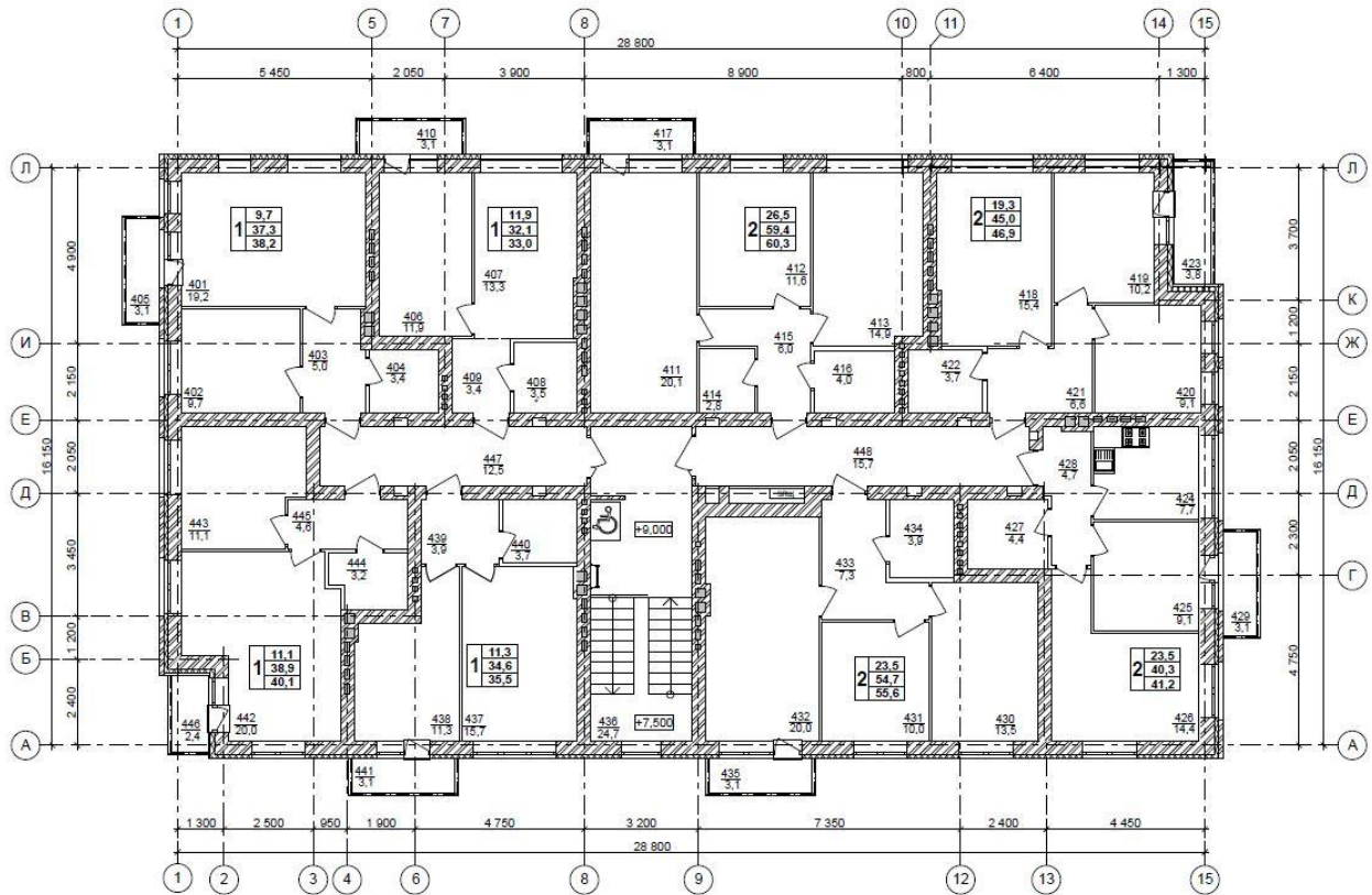
План 4 этажа
