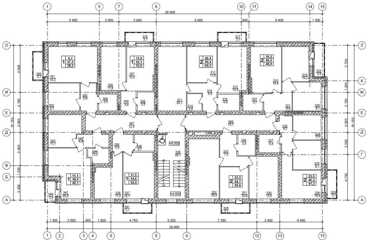
План 3 этажа
